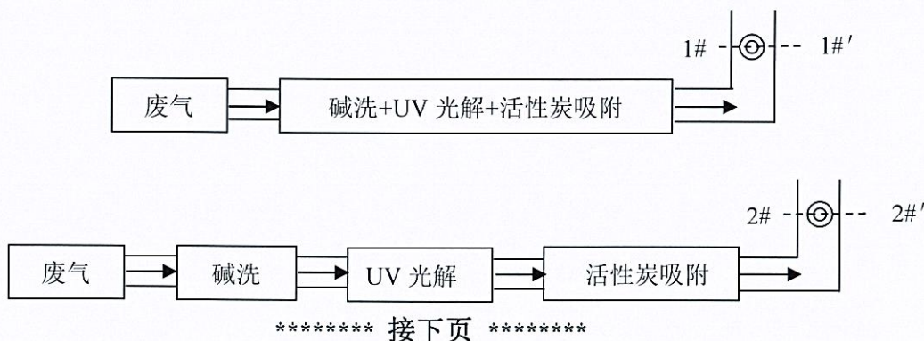
废气处理工艺流程图
