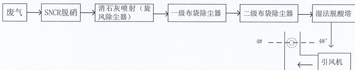
废气处理工艺流程图
