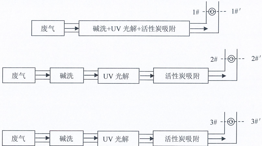
废气处理工艺流程图
